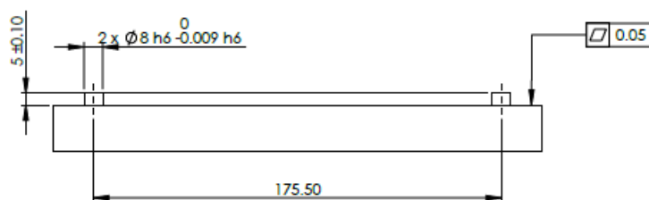
1.2: 機器人底座安裝板
